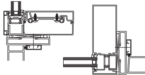
Door Details
